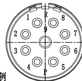
针位排布图
