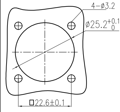
面板开孔图
