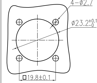
面板开孔图
