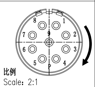
针位排布图
