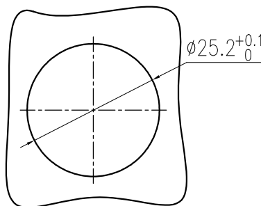
面板开孔图
