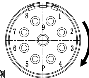
针位排布图
