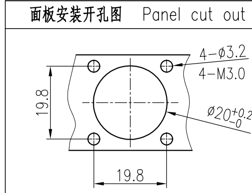
比例 Scale: 2:1
