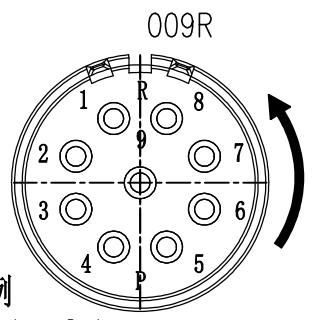
比例 Scale: 2:1
