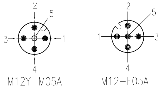
孔位示意图
