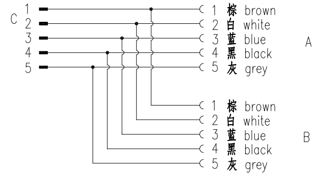
线路图
