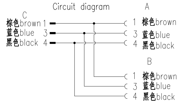
接线图
