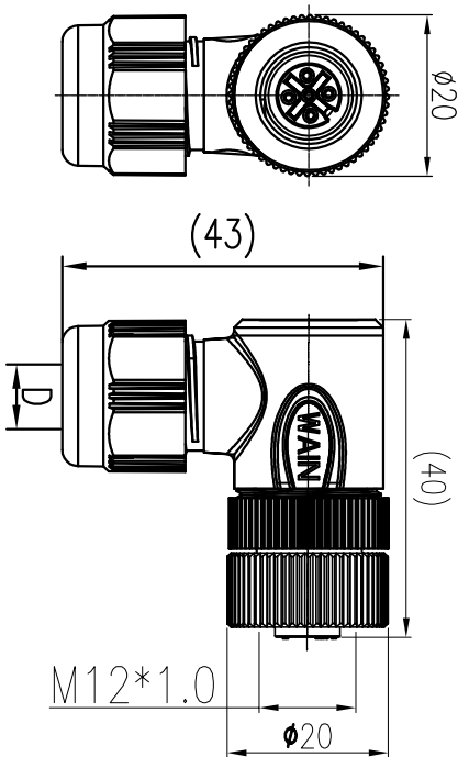
电缆直径:D6,D8 Cable outlet:D6,D8
