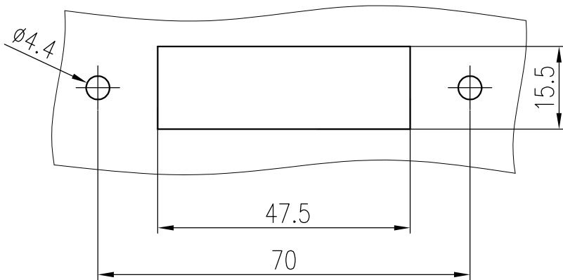
面板开孔图
