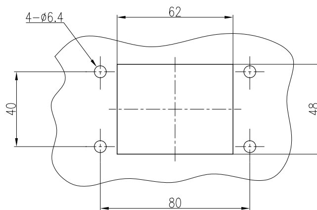
面板开孔图
