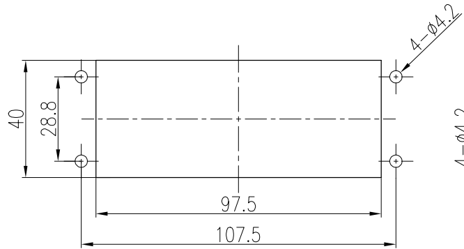
开孔尺寸图 (Paenl cut out)
