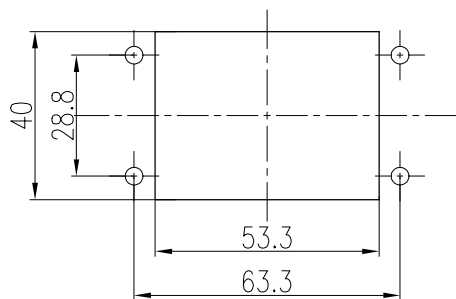
开孔尺寸图 (Paenl cut out)
