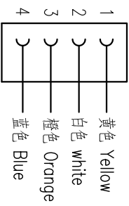
接线图 Circuit diagram
